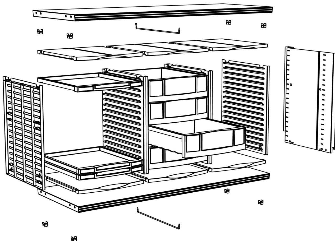
Vue Eclatée
